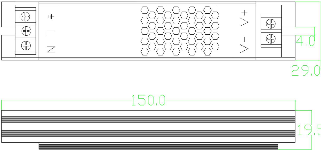
端子台脚位定义
