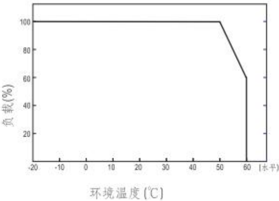
衰减曲线
